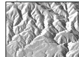
Modelos Dixitais de Elevacións (MDE)
